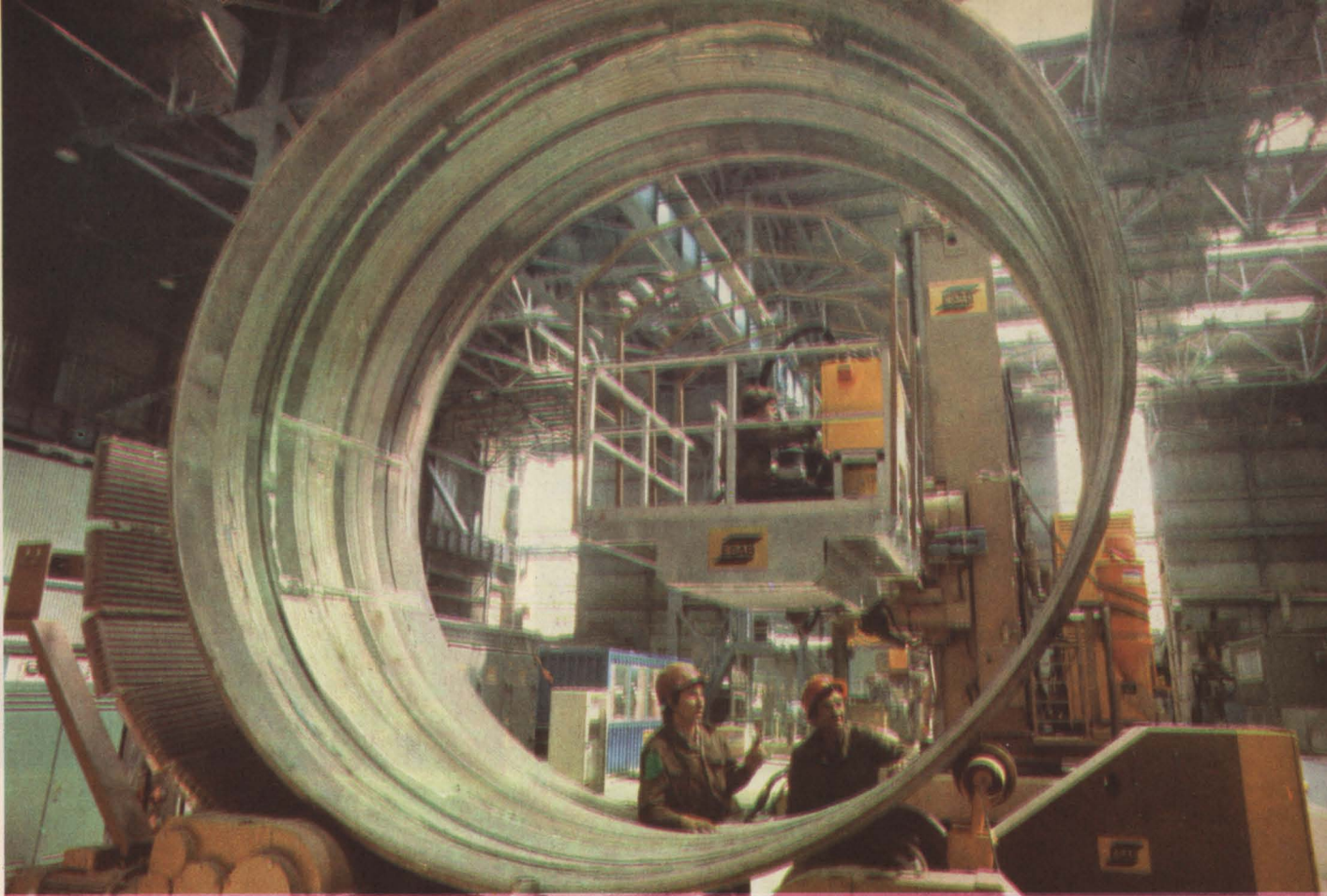
Атоммаш. Сварочные работы на корпусе атомного реактора.
